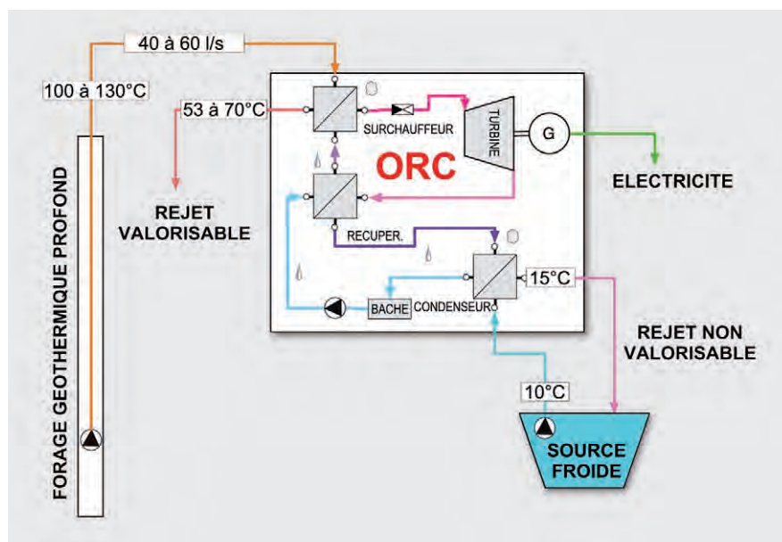
Figure 1 Schéma simplifié du fonctionnement d'un forage géothermique profond.
